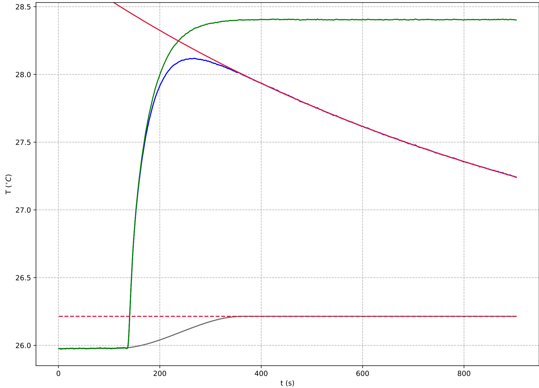
Fajhő mérése beejtéssel
