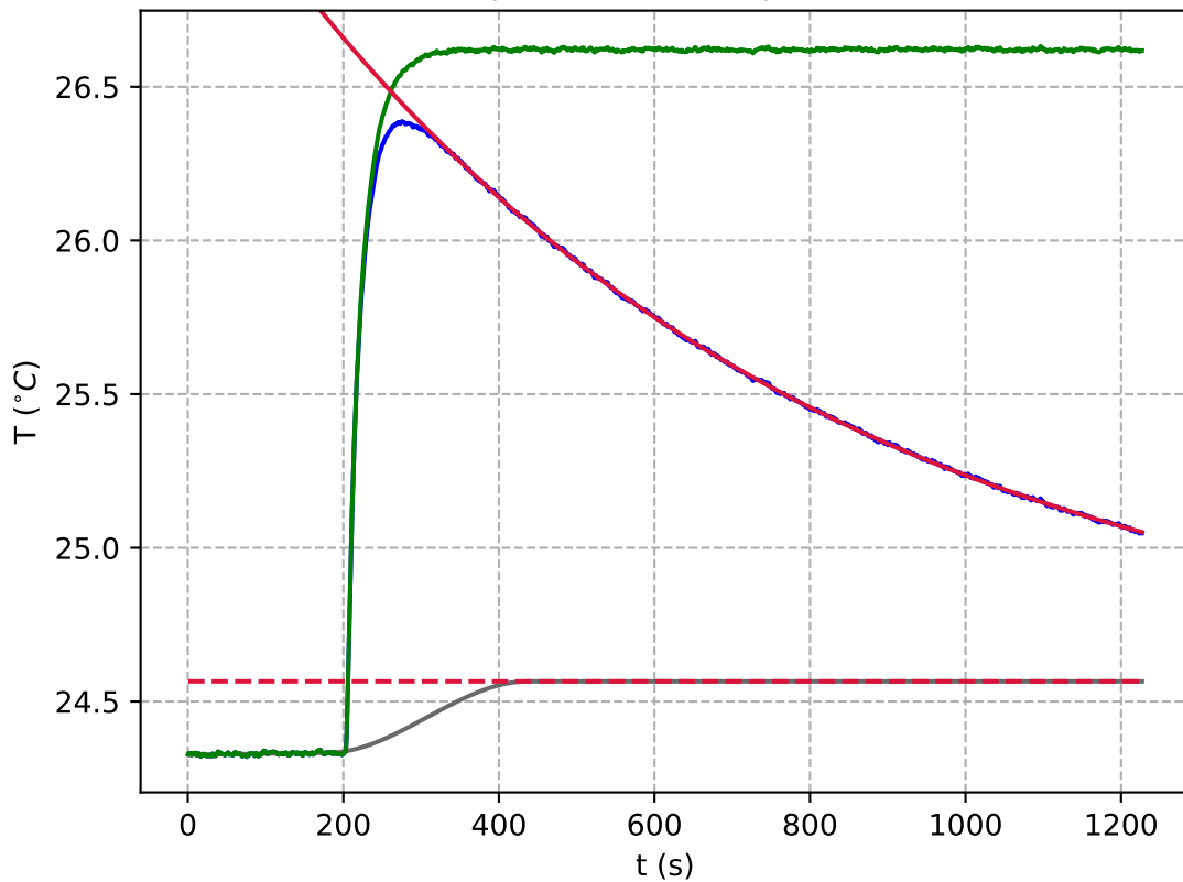
Fajhő mérése beejtéssel
