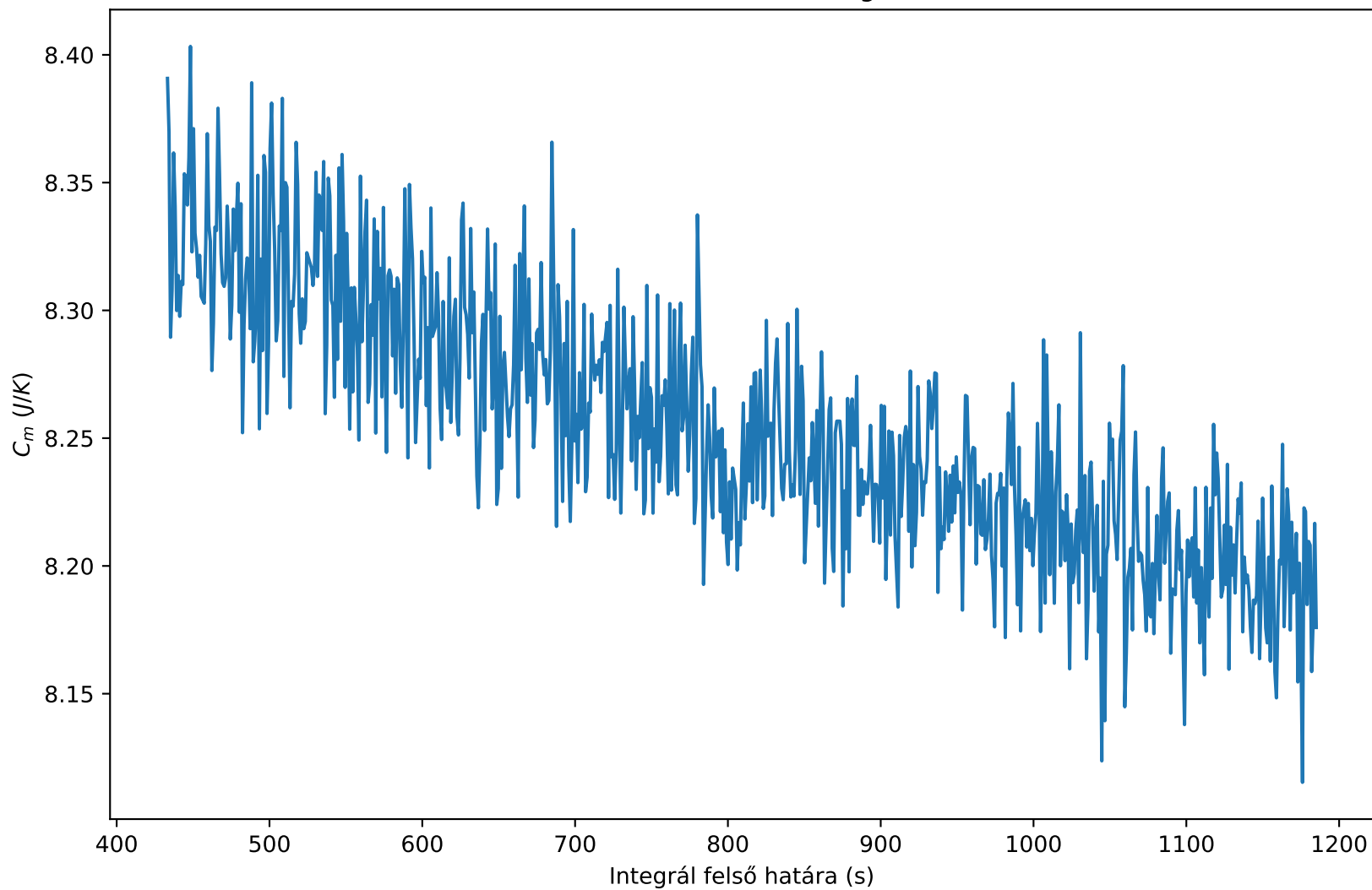
Variált felső határú integrálás
