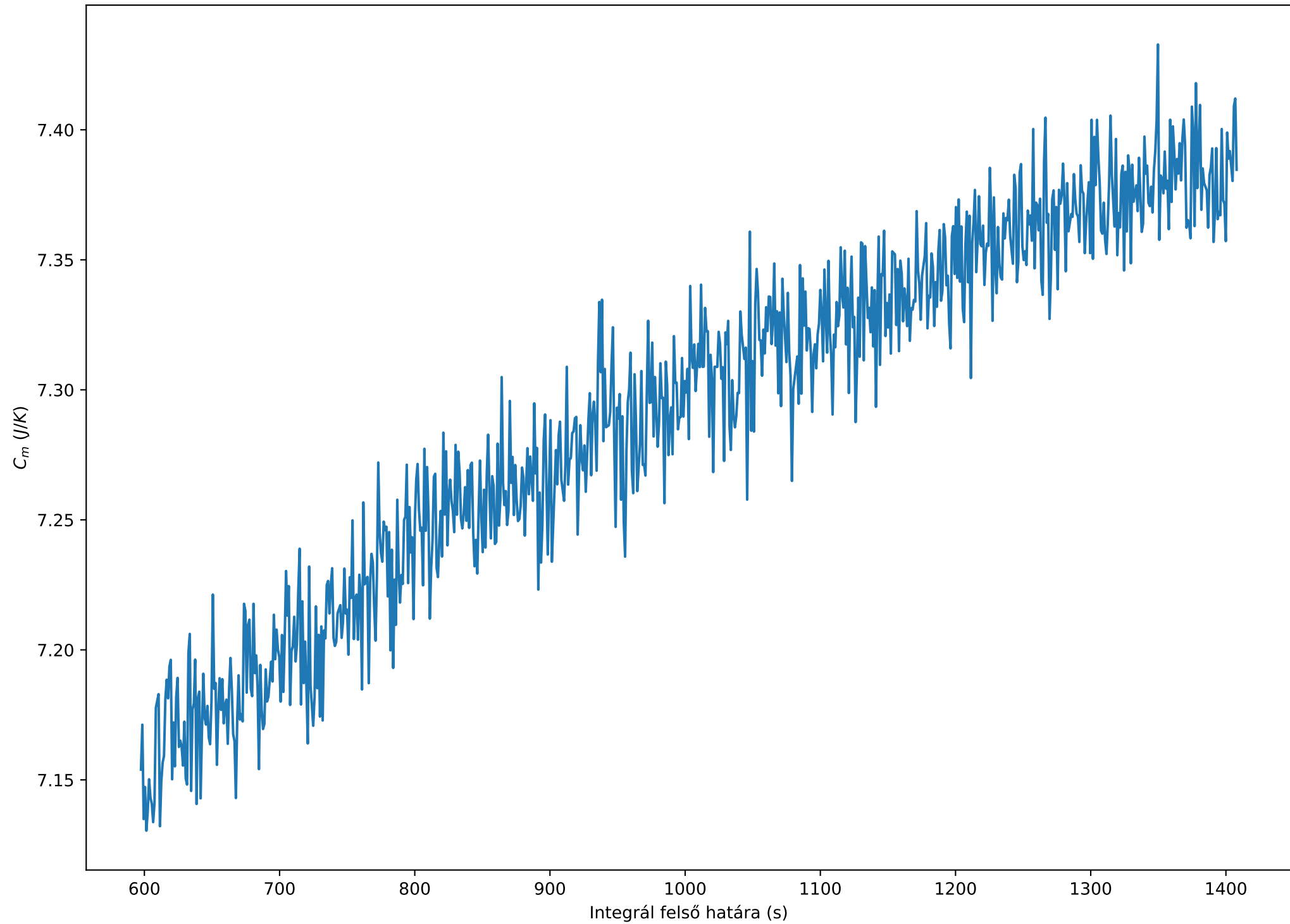
Variált felső határú integrálás
